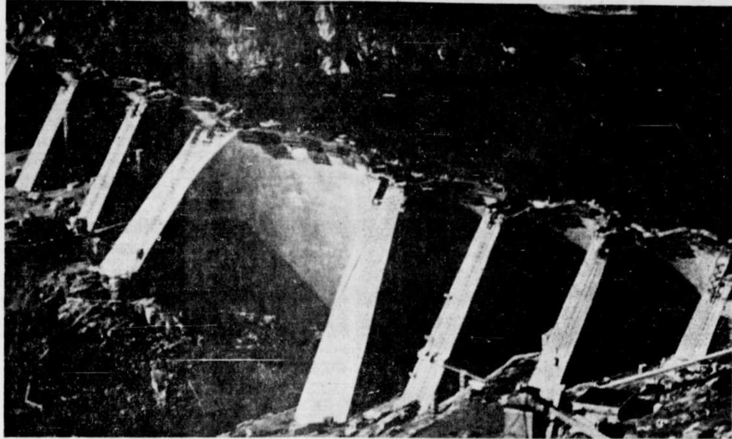
● Le principal ouvrage du complexe hydro-électrique de Manicouagan - Aux-Outardes est sans contredit le barrage de Manic 5 qui constitue le plus grand barrage à arches multiples au monde. Les dernières couches de ciment seront coulées ce printemps au sommet de l'arche principale et des treize arches latérales qui s'étendent sur 4,310 pieds à travers la vallée.
